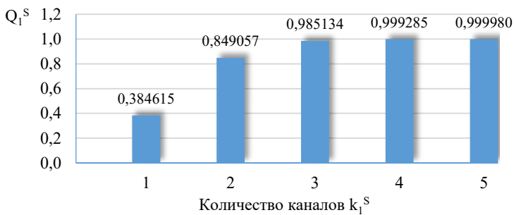
Рис. 5. Зависимость относительной пропускной способности Q_1^S от количества каналов 1-го узла подсистемы S
